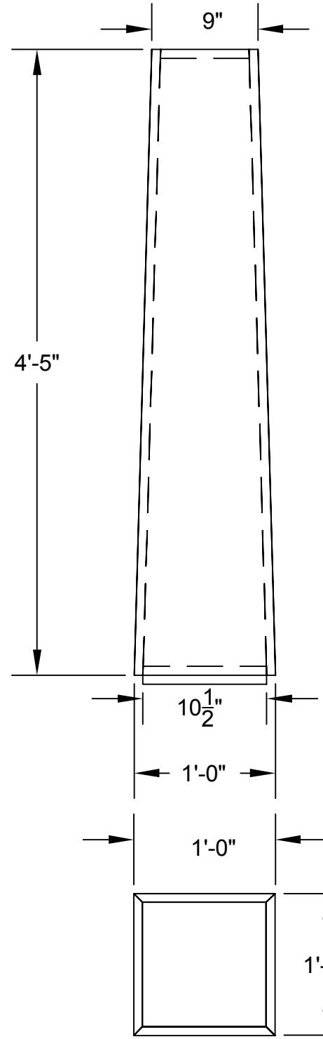
COLUMN TOP SCALE: 1"=1'-0"
